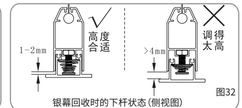
银幕回收时的下杆状态(侧视图)
